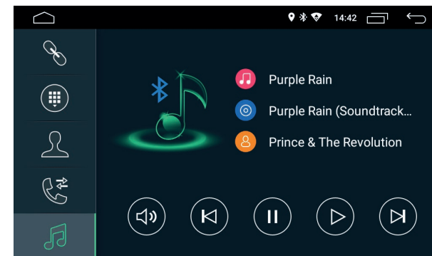
Приложение Bluetooth-музыка
